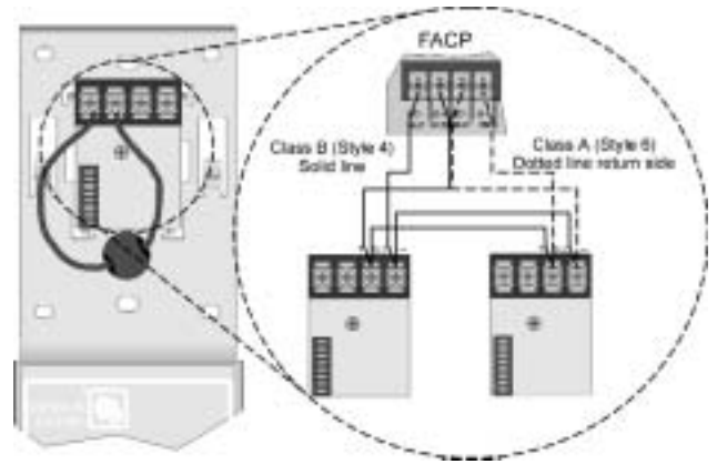
SLC Wiring
